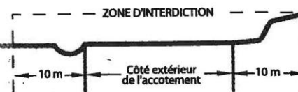
ROUTE STANDARD AVEC UN FOSSE ET UN ESCARPEMENT
